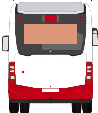
Achterraam (1600 x 600 mm)
