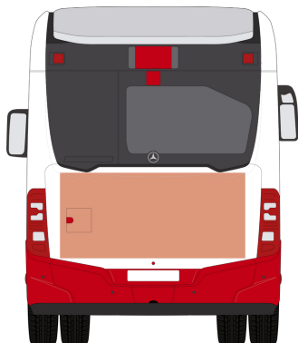
Achterklep (1850 x 850 mm)
